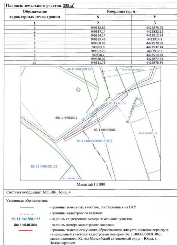
Схема границ сервитута на кадастровом плане территории
