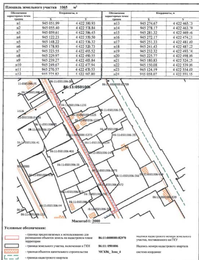
Схема границ сервитута на кадастровом плане территории
