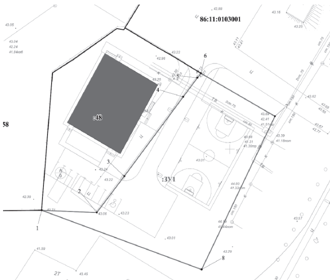
Чертеж образования земельного участка (I этап)
