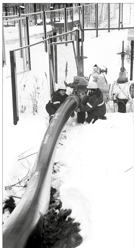
Байпас – временная линия, по которой осуществляют запуск нефтесодержащей эмульсии.
