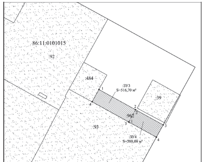
Чертеж образования земельных участков :ЗУ3 и :ЗУ4 (II этап) (раздел земельного участка с кадастровым номером 86:11:0101015:962)
