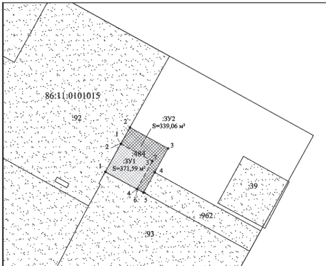
Чертеж образования земельных участков :ЗУ1 и :ЗУ2 (I этап) (раздел земельного участка с кадастровым номером 86:11:0101015:484)
